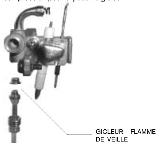
Fig. 13 - Dispositif de la flamme de veille
