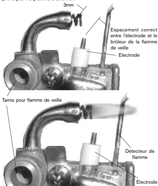
Fig. 12 - Flamme de veilleuse typique
