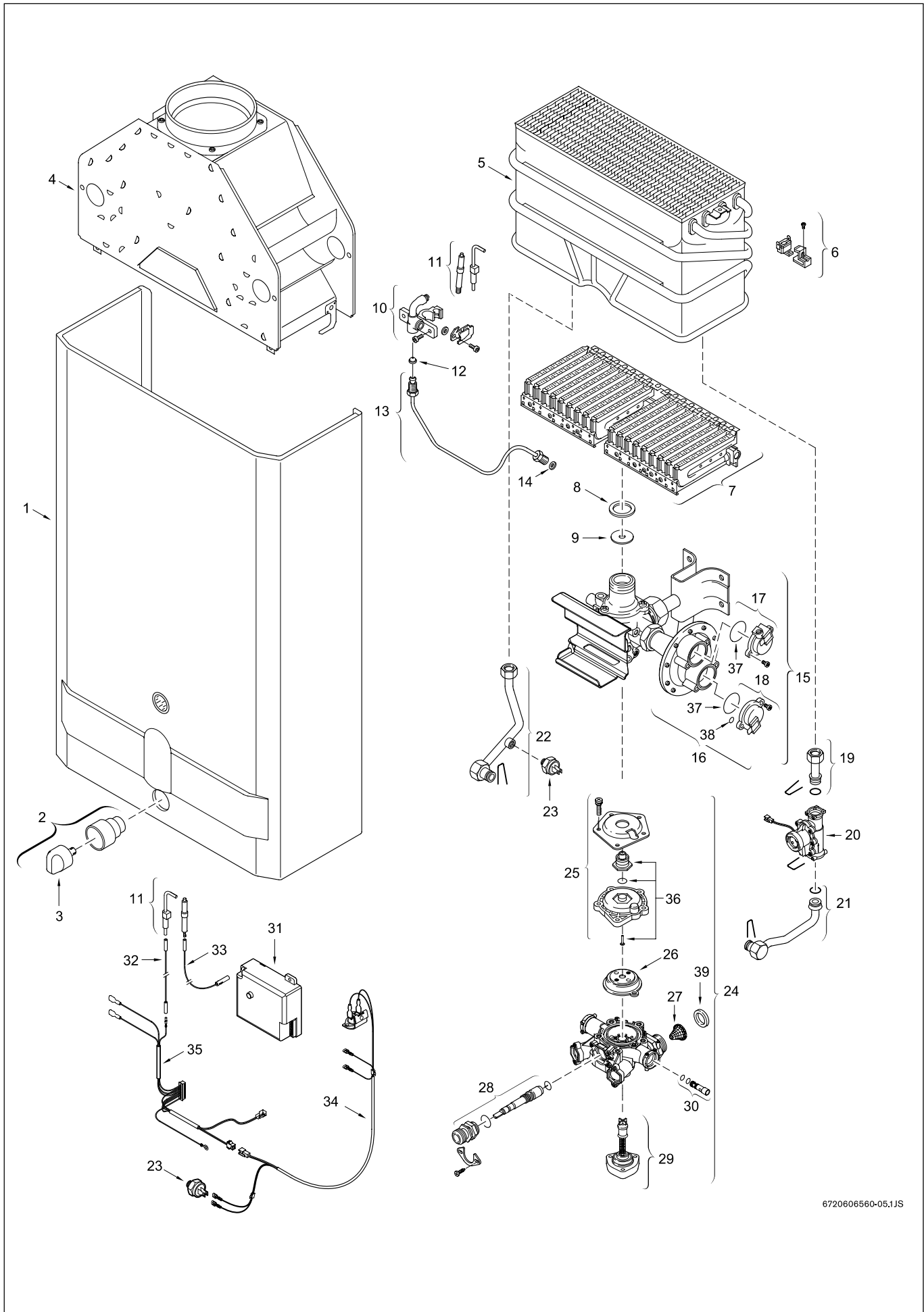
Fig. 16 - COMPOSANTS INTERNES DU CHAUFFE-EAU WR 400-7.K.. ET LISTE DES PIÈCES
