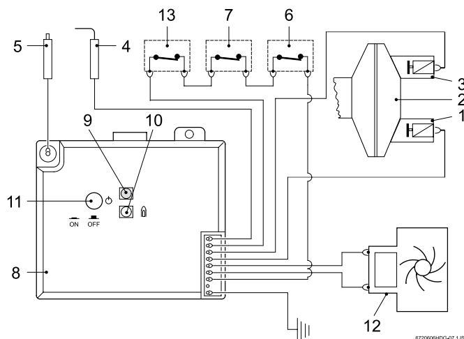
Fig. 14 - Schéma des circuits électriques
